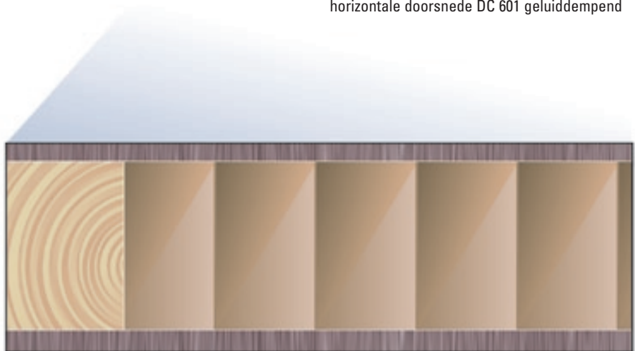
horizontale doorsnede D 601
