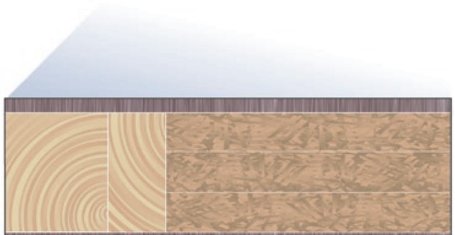
horizontale doorsnede DC 601 geluiddempend
